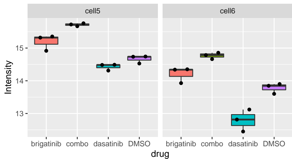
Ctnnd1_T869
