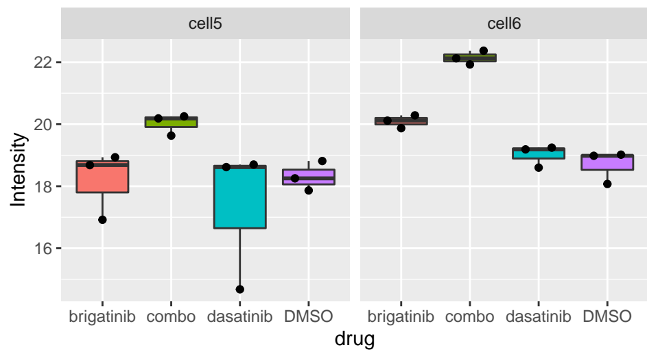
Dek_S312
