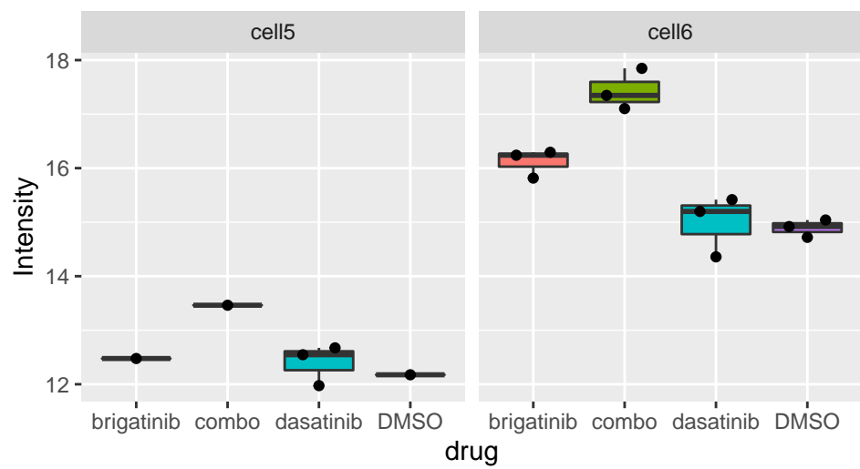
Son_S1807
