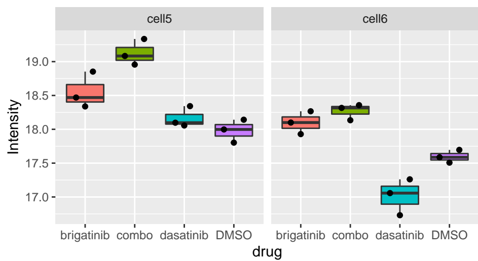
Abcc5_S505
