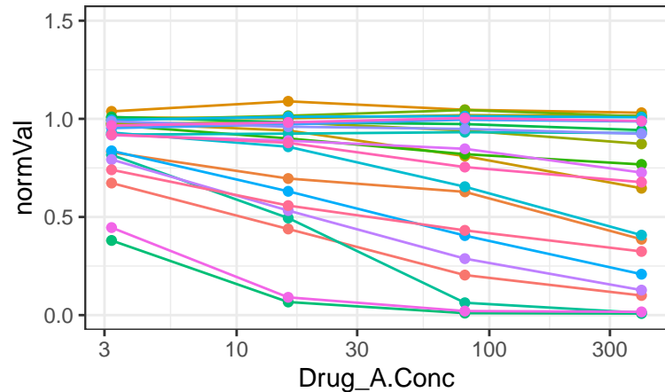
Venetoclax_DMSO_0
