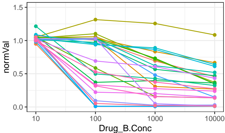
V-9302
