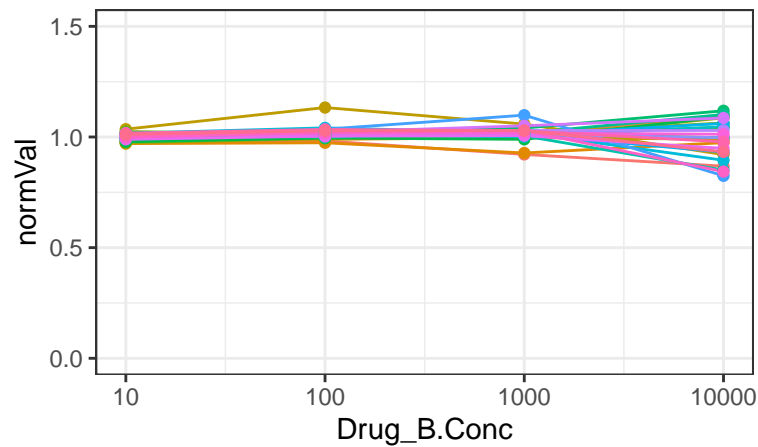
Thiomyristoyl
