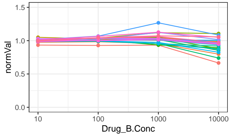
BT2
