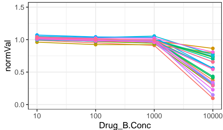
Firsocostat
