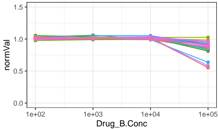
Etomoxir
