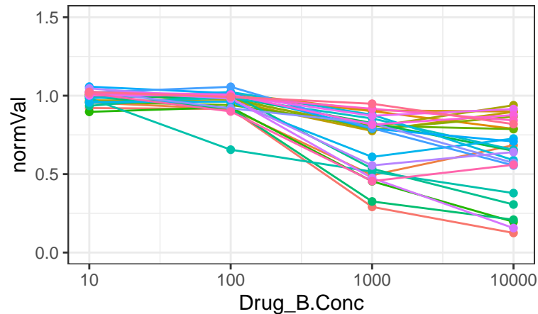
CPI-613
