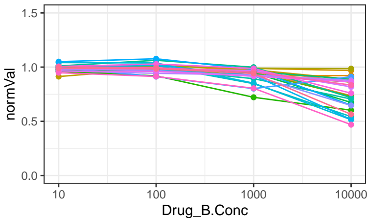
SHIN1
