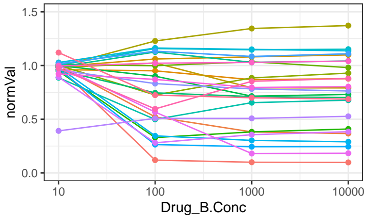
AZD3965
