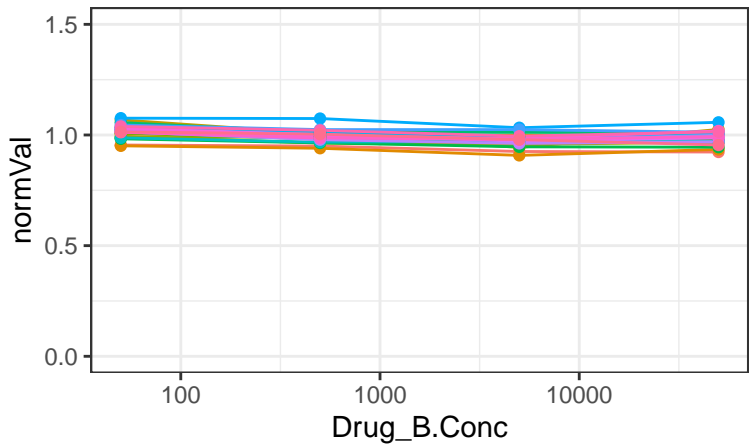
Selisistat
