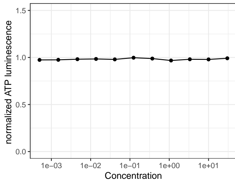
Ebselen
