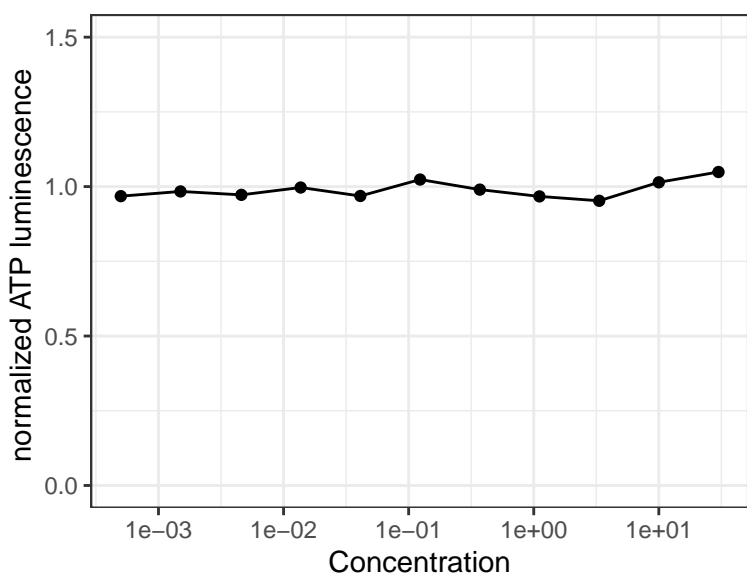
Dasatinib
