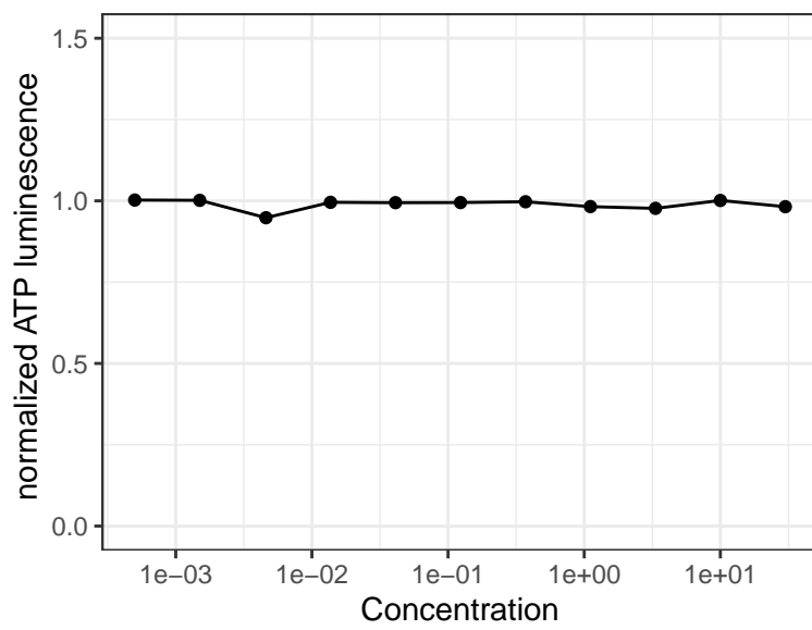
PKI-402
