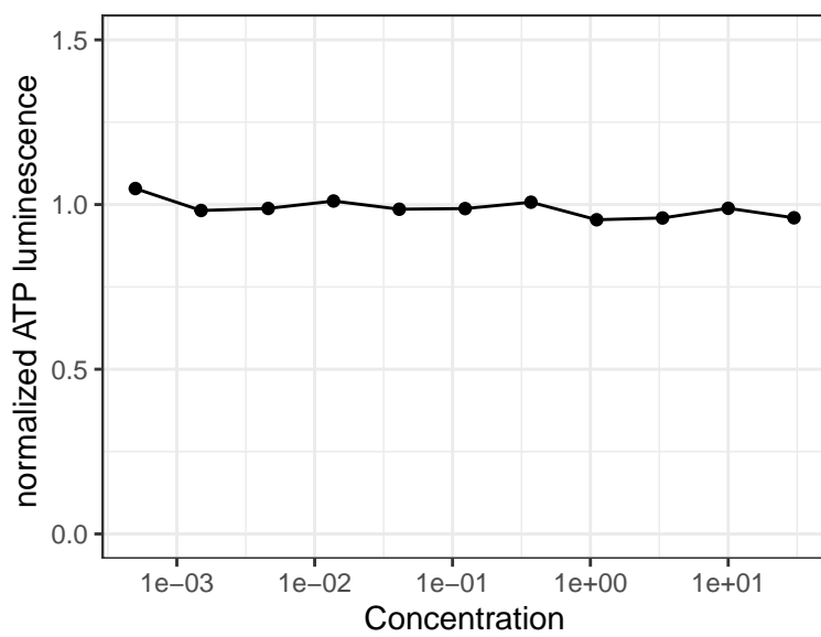
Odanacatib
