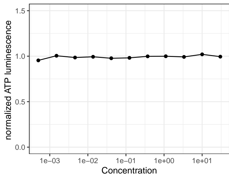
MLN9708
