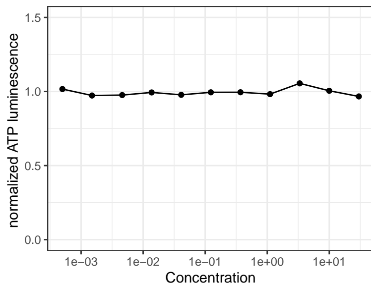
CTA056
