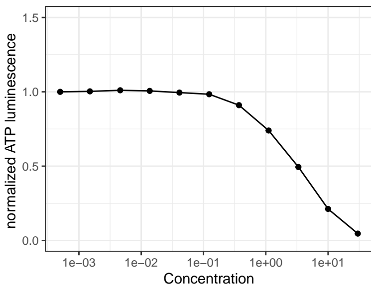
10058-F4
