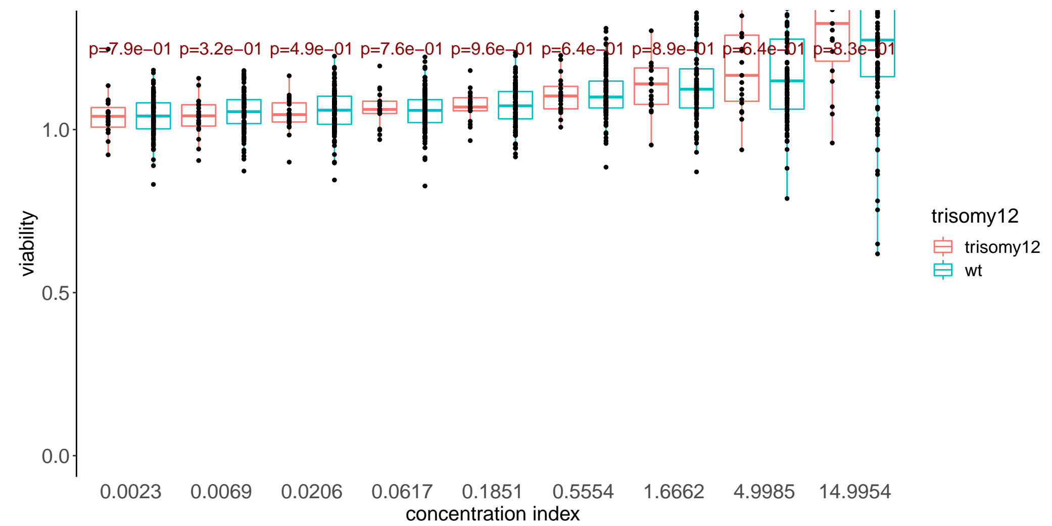
QS11
