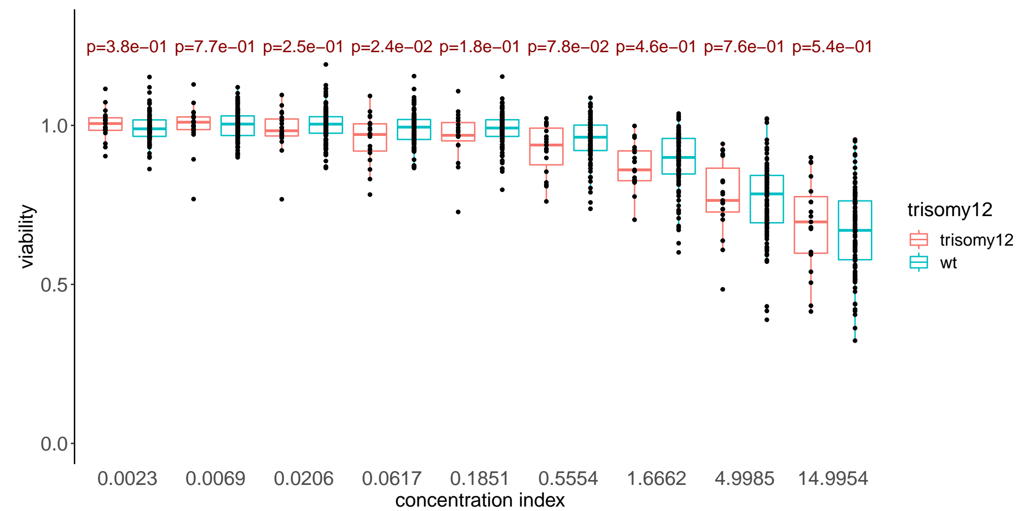
Enzastaurin
