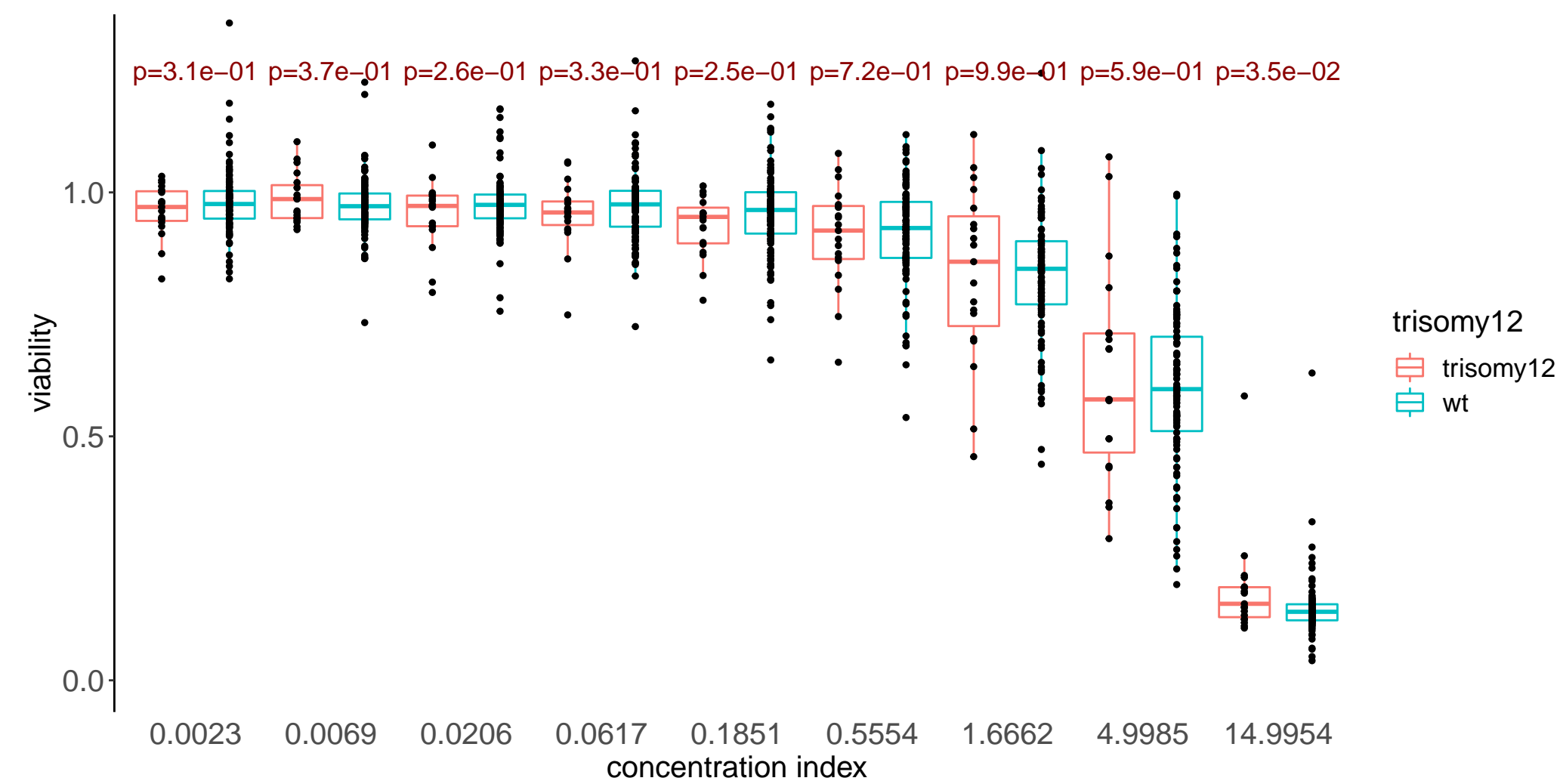
Ceritinib
