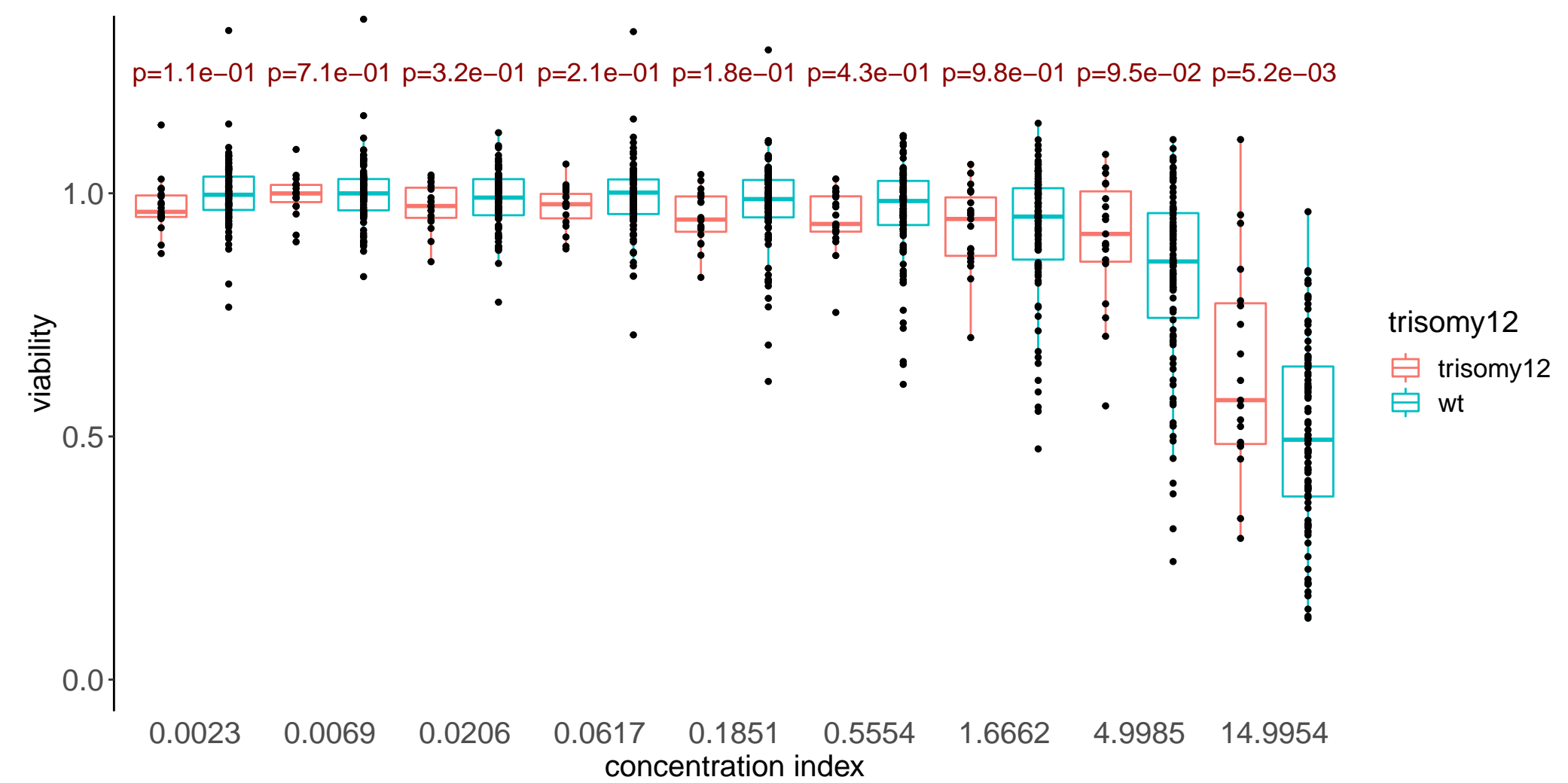
KN-93
