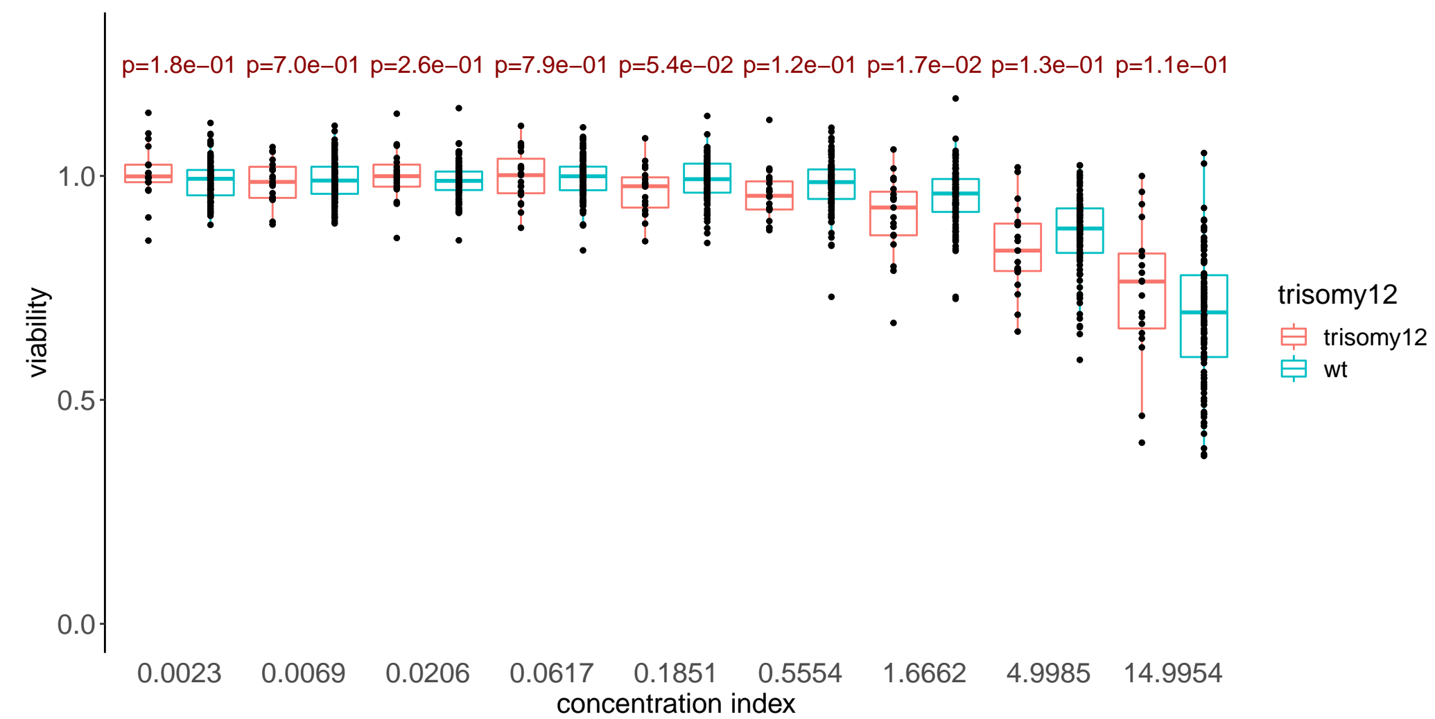
Roscovitine
