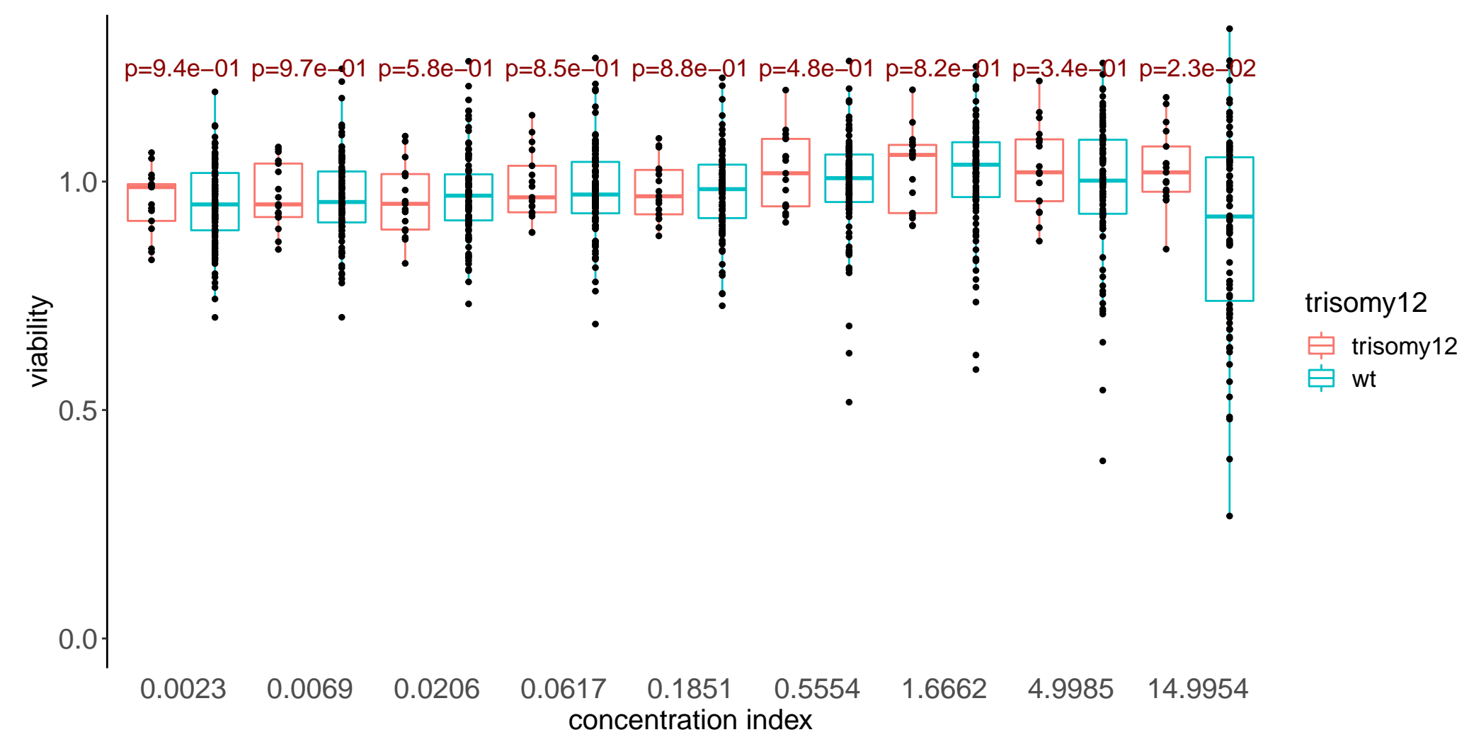
SirReal2
