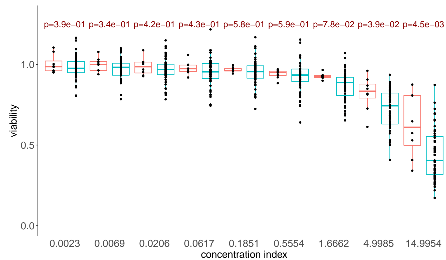
Nexturastat A
