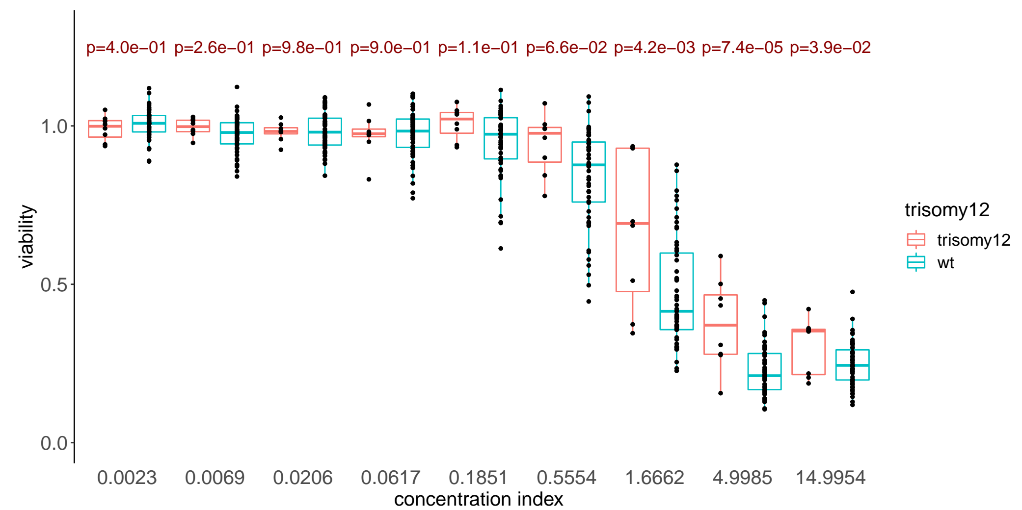
Resminostat
