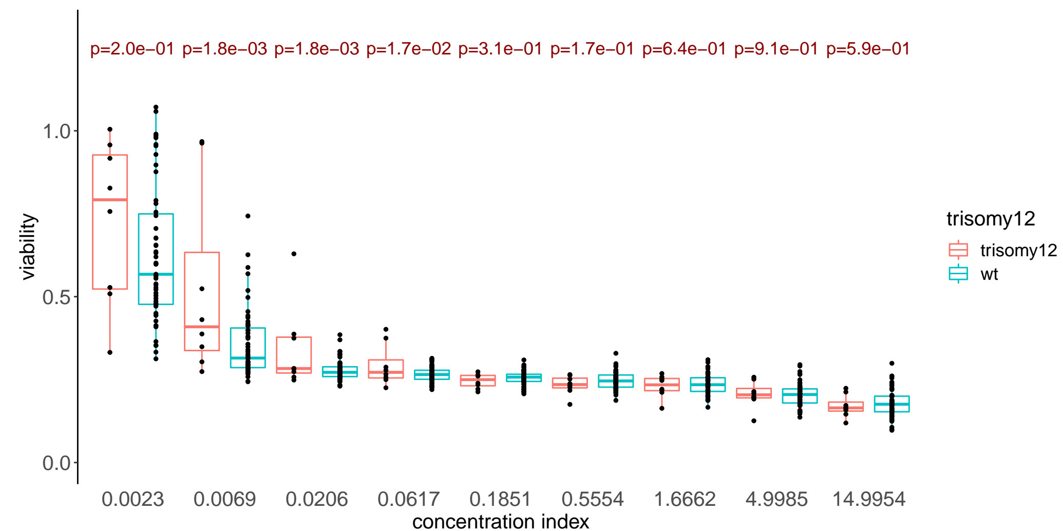
Carfilzomib
