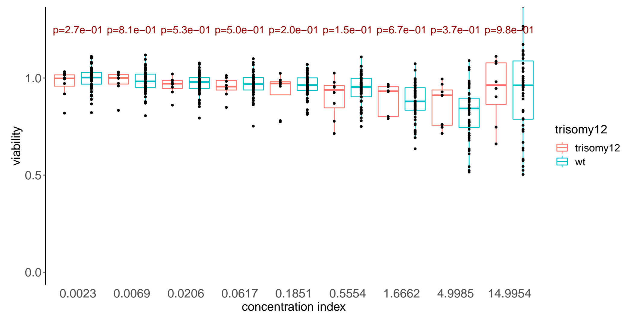
RAF265
