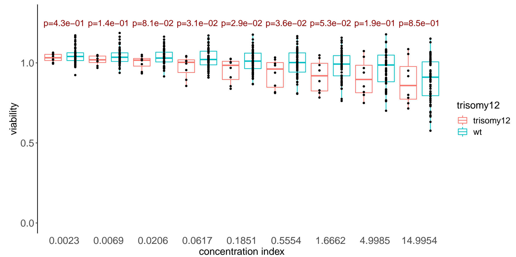
Selumetinib
