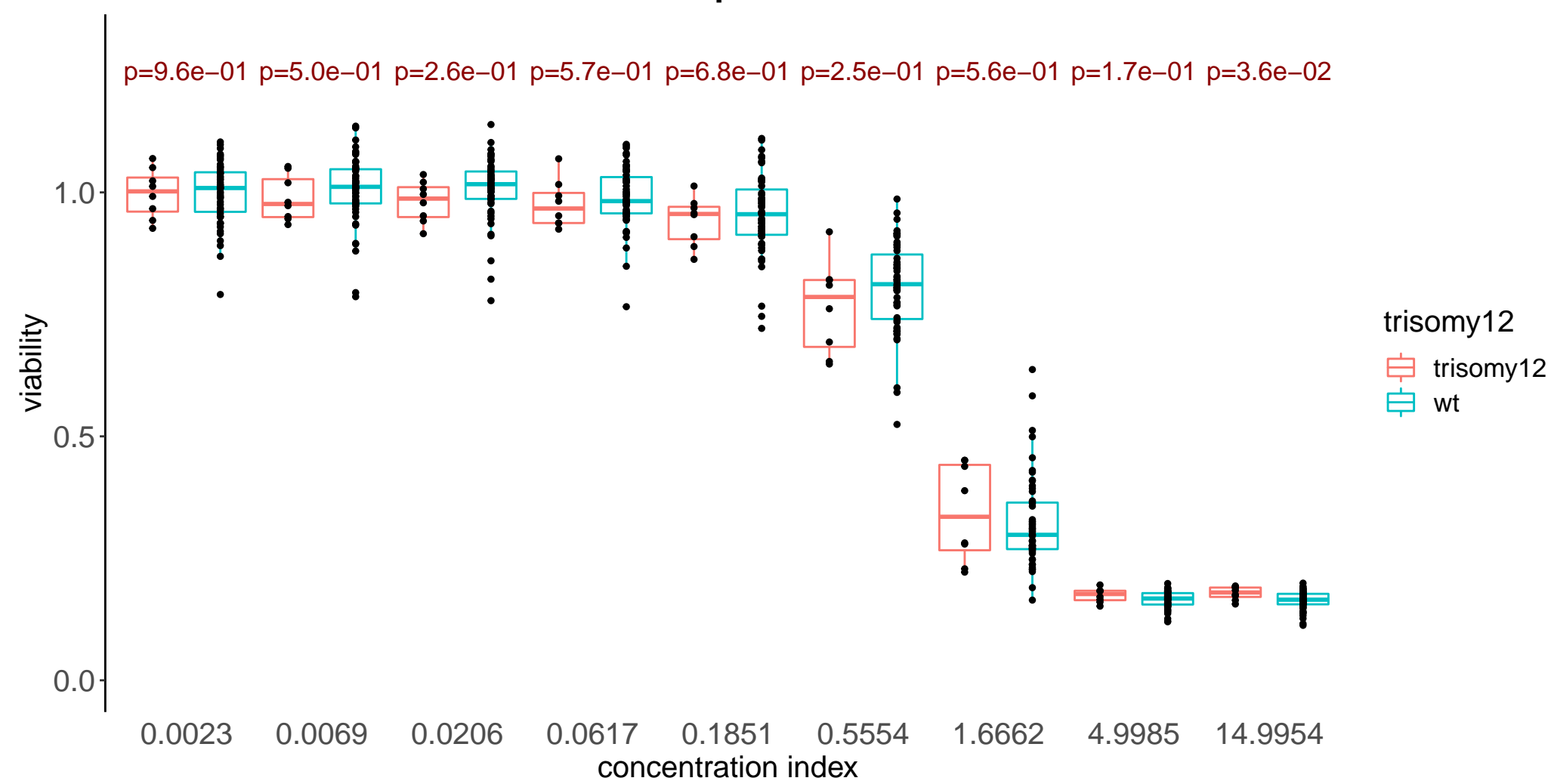
Entospletinib
