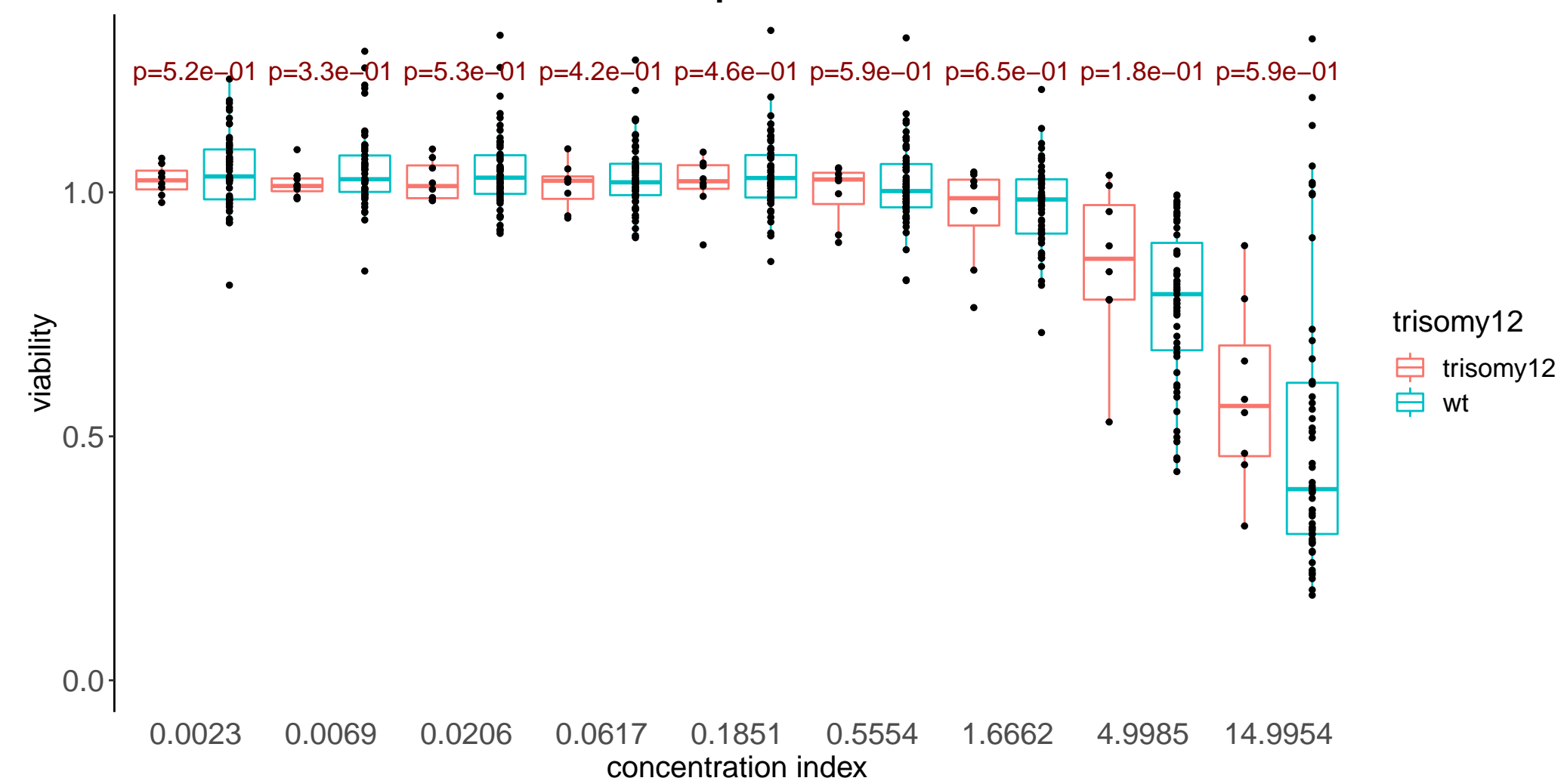
Iniparib
