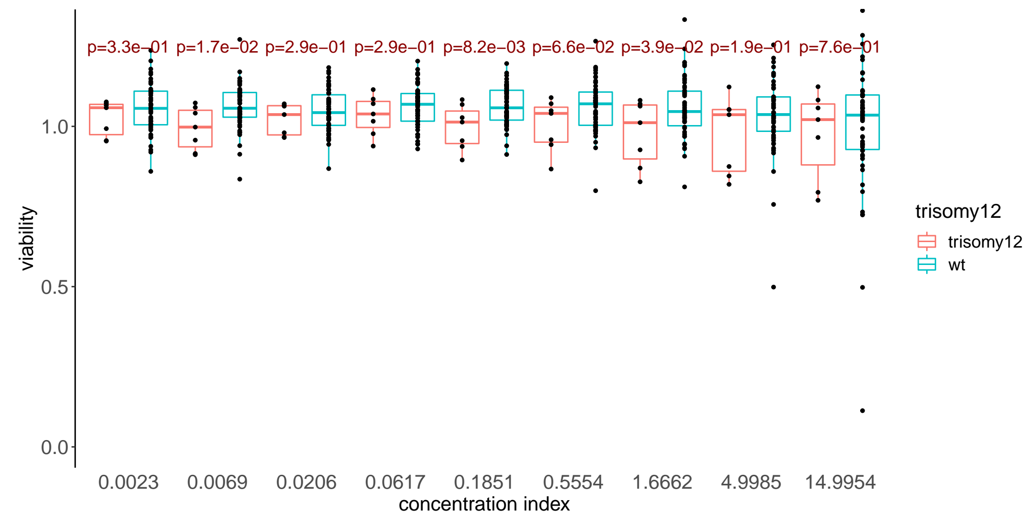
Plerixafor
