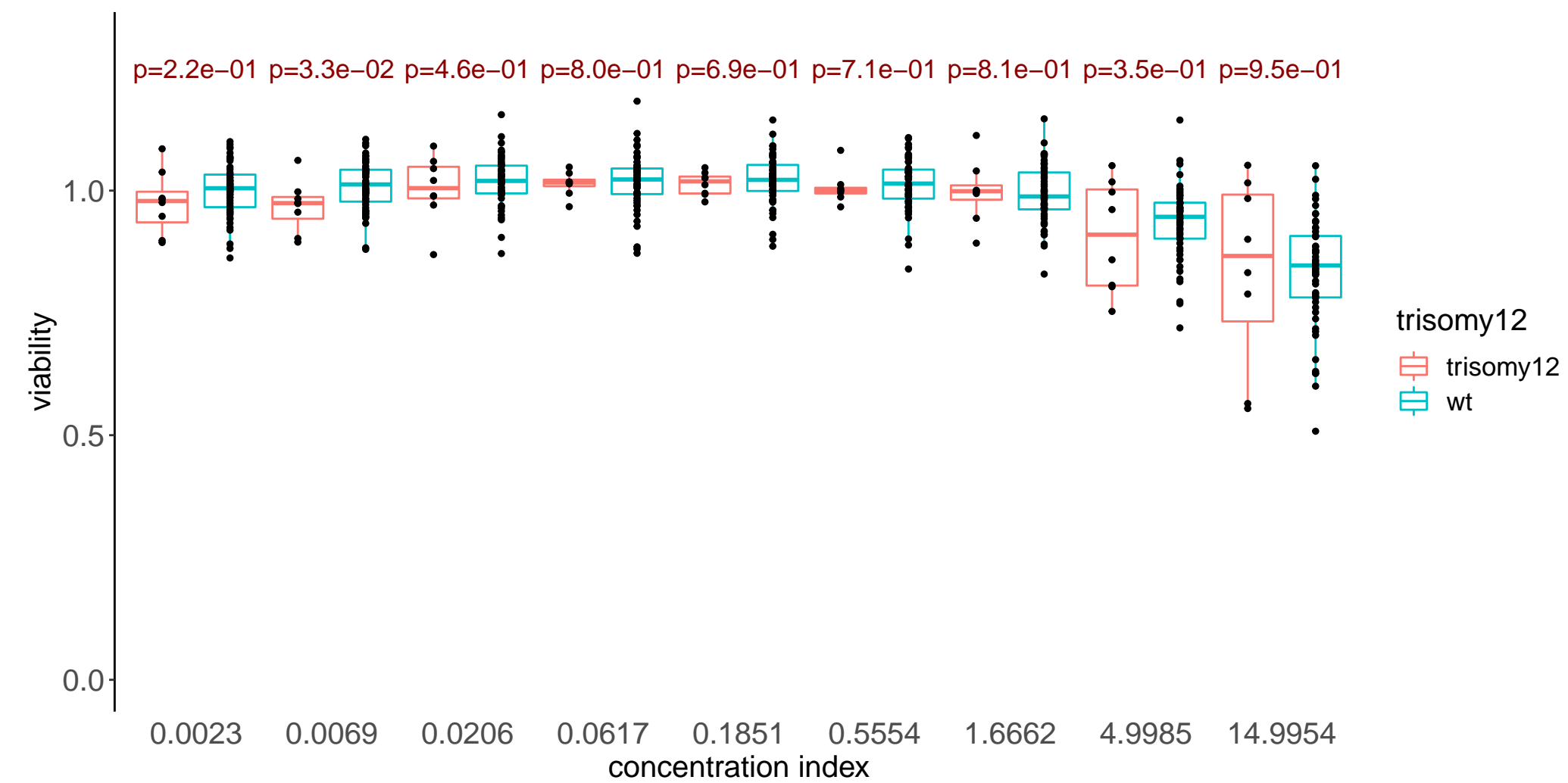
Dabrafenib
