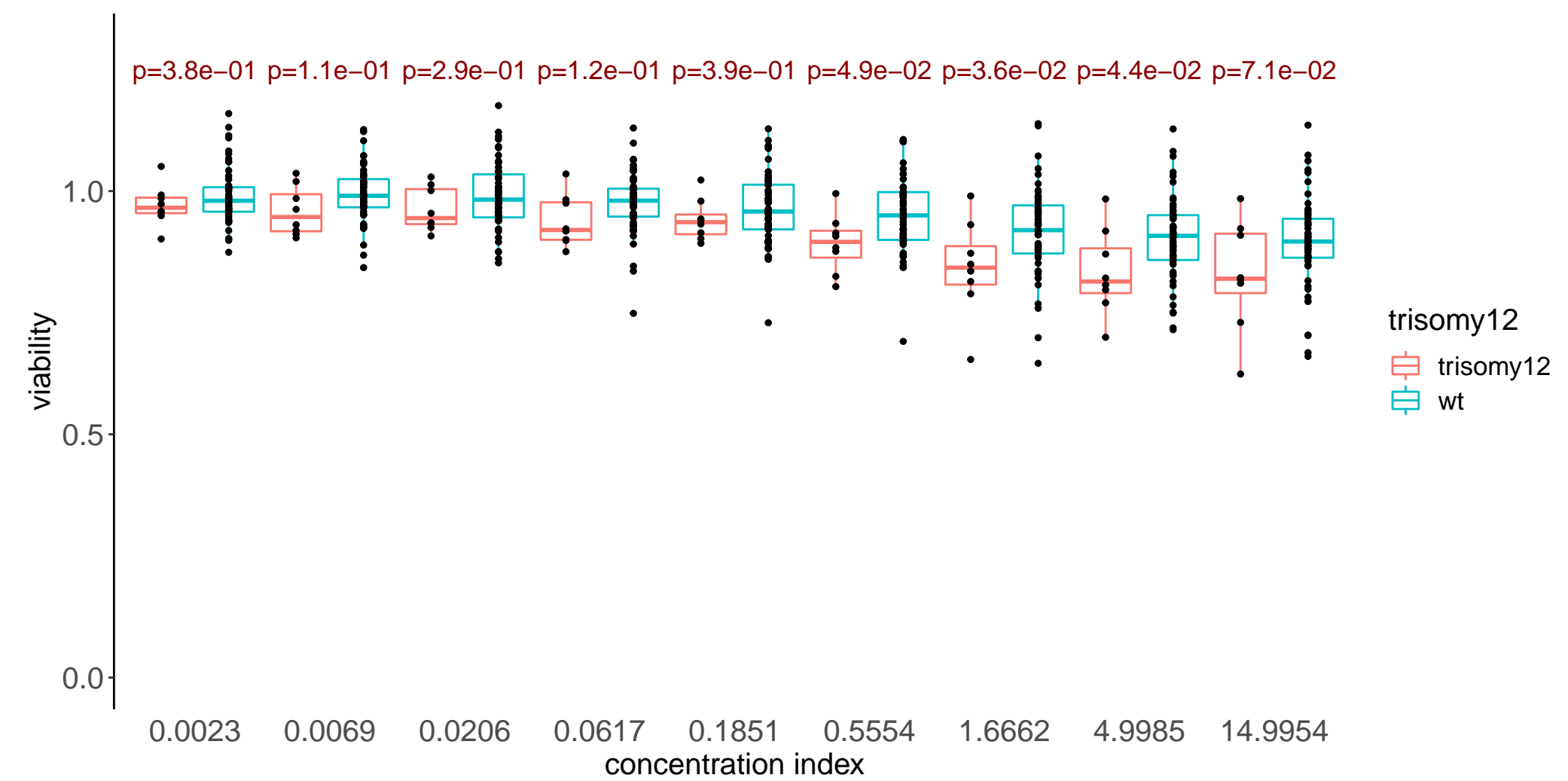
R406
