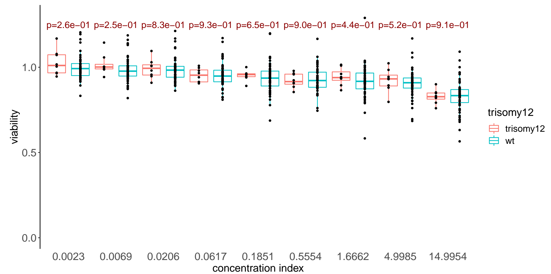
LY2584702
