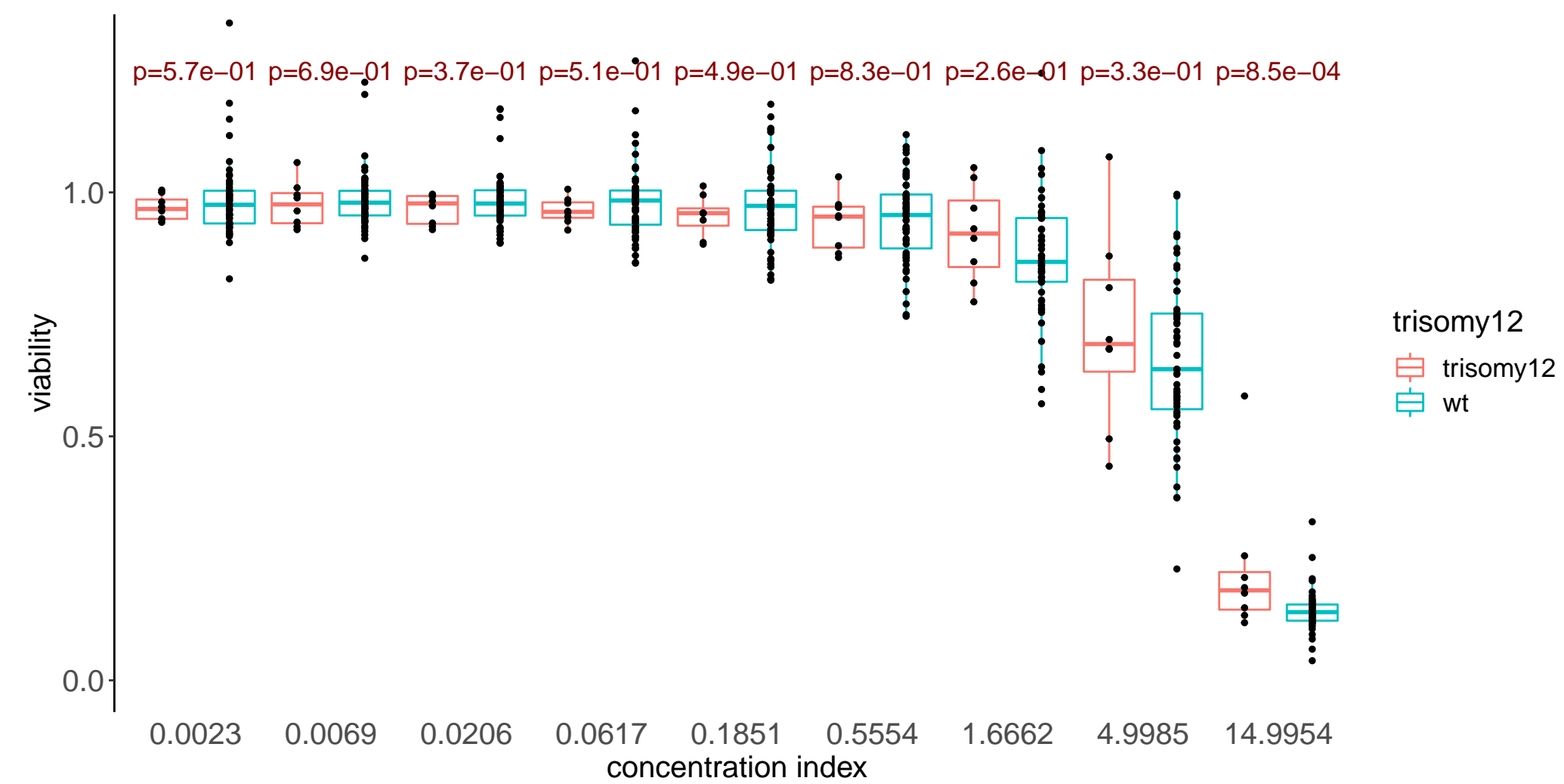
Ceritinib
