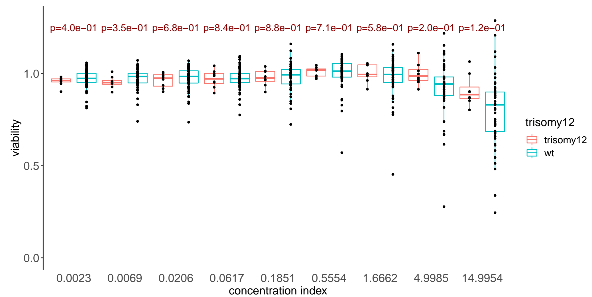
ICG-001
