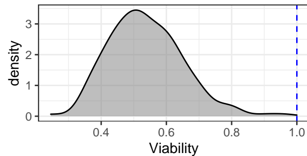
SGI-1776
