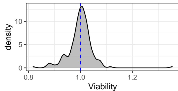
EW-7197
