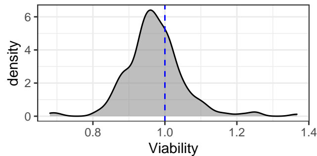
GSK2801
