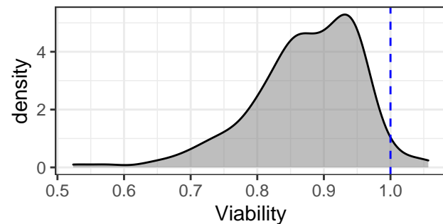
EW-7197
