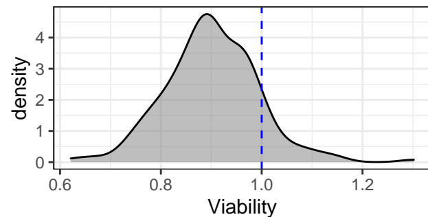
Ro-3306
