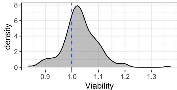
Temsirolimus
