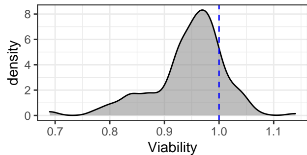
z-LVSR-fmk
