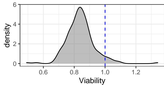
Nifuroxazide
