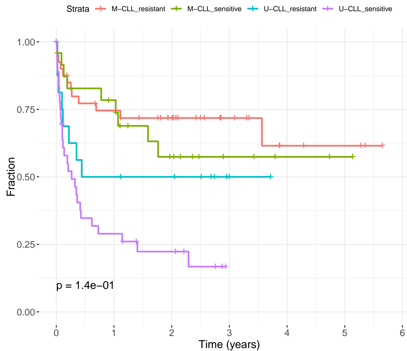
JNK-IN-8~ TTT
