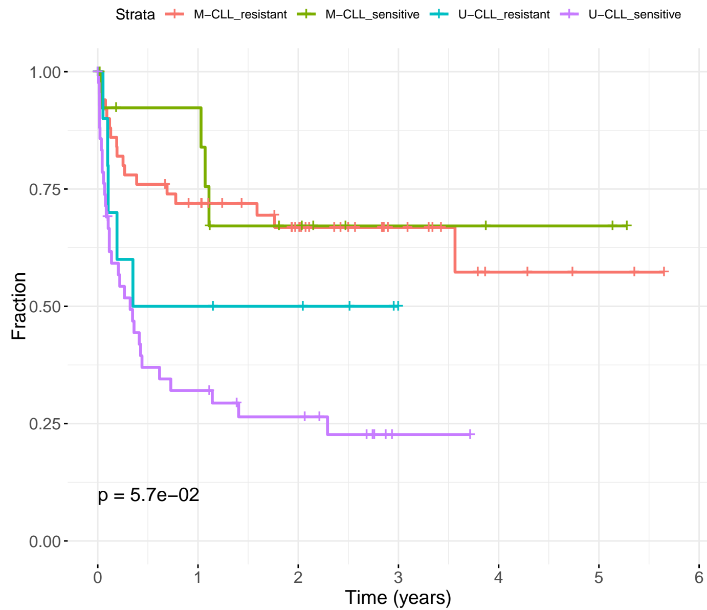
Ponatinib~ TTT
