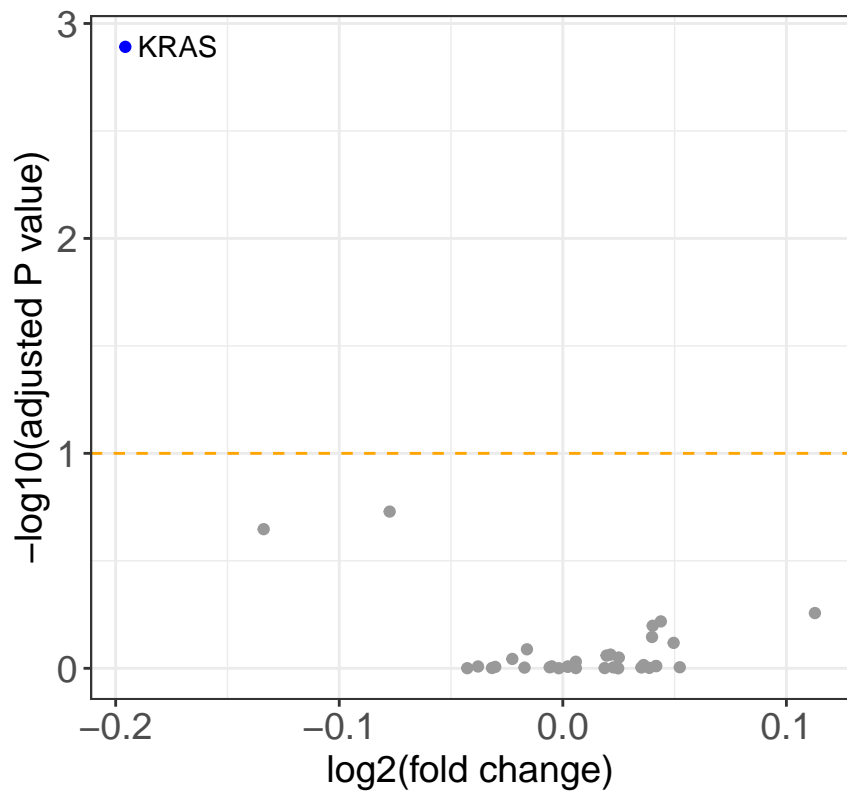
SCH772984
