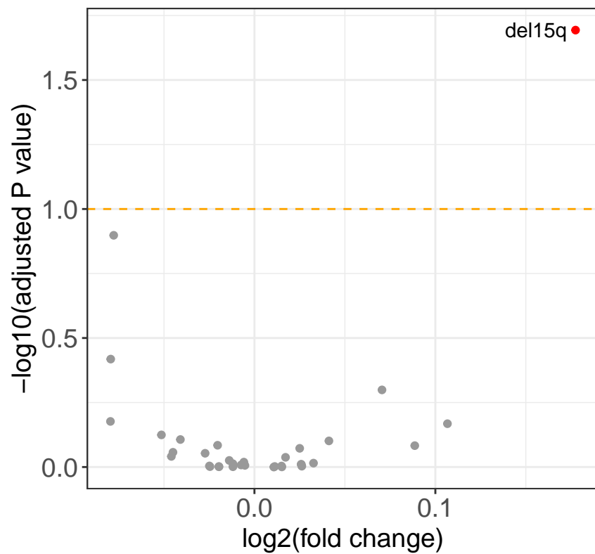
CAY10603
