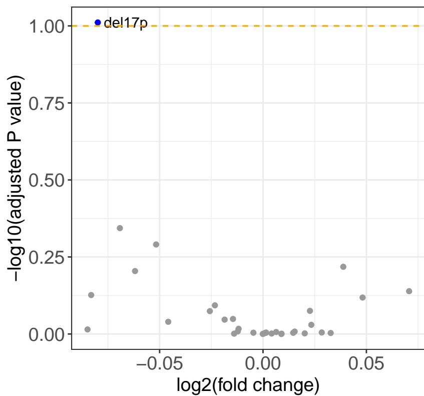
z-LVSR-fmk
