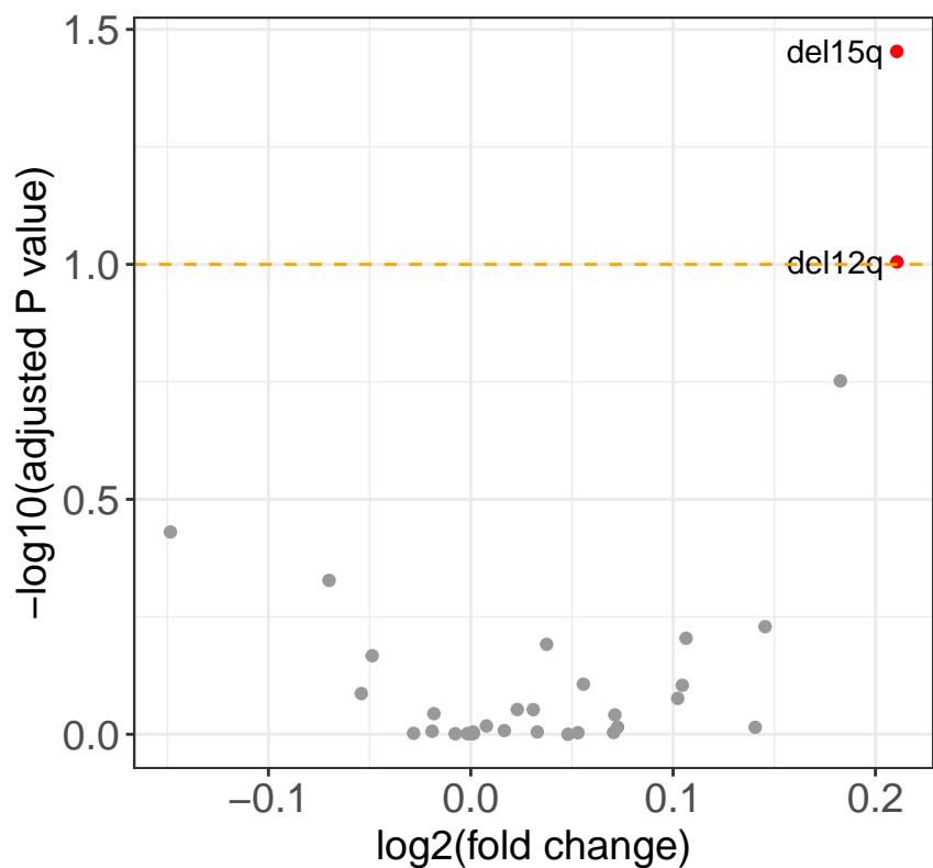
RKI-1447
